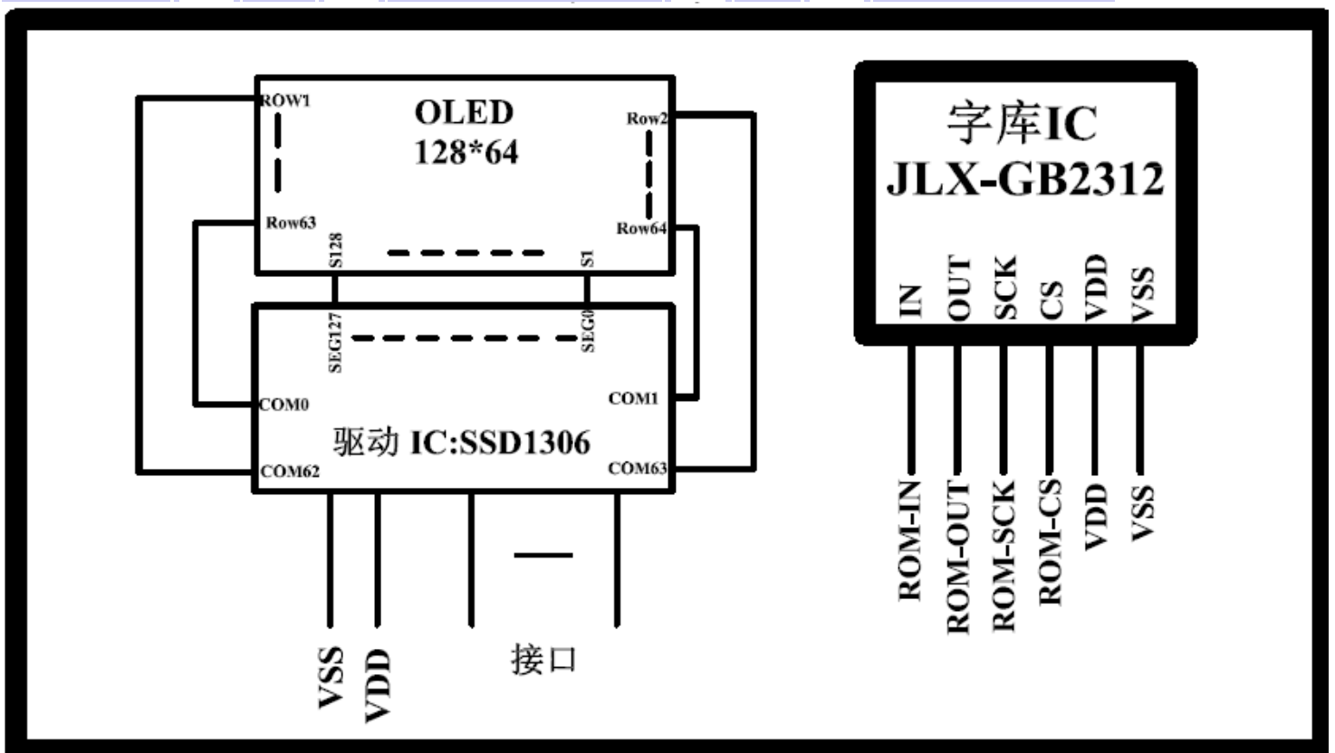
图 2. JLX12864OLED-096
