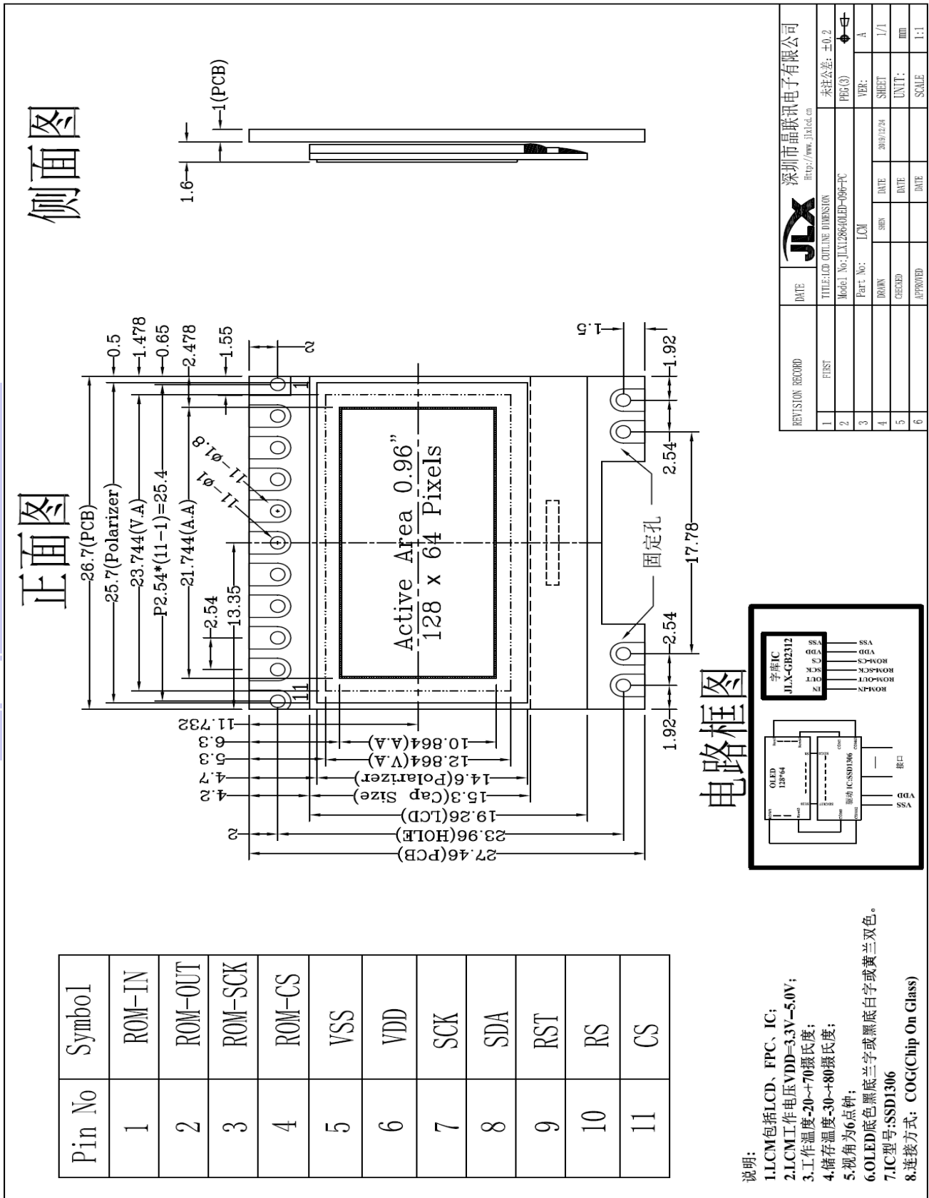
图 1. 外形尺寸
