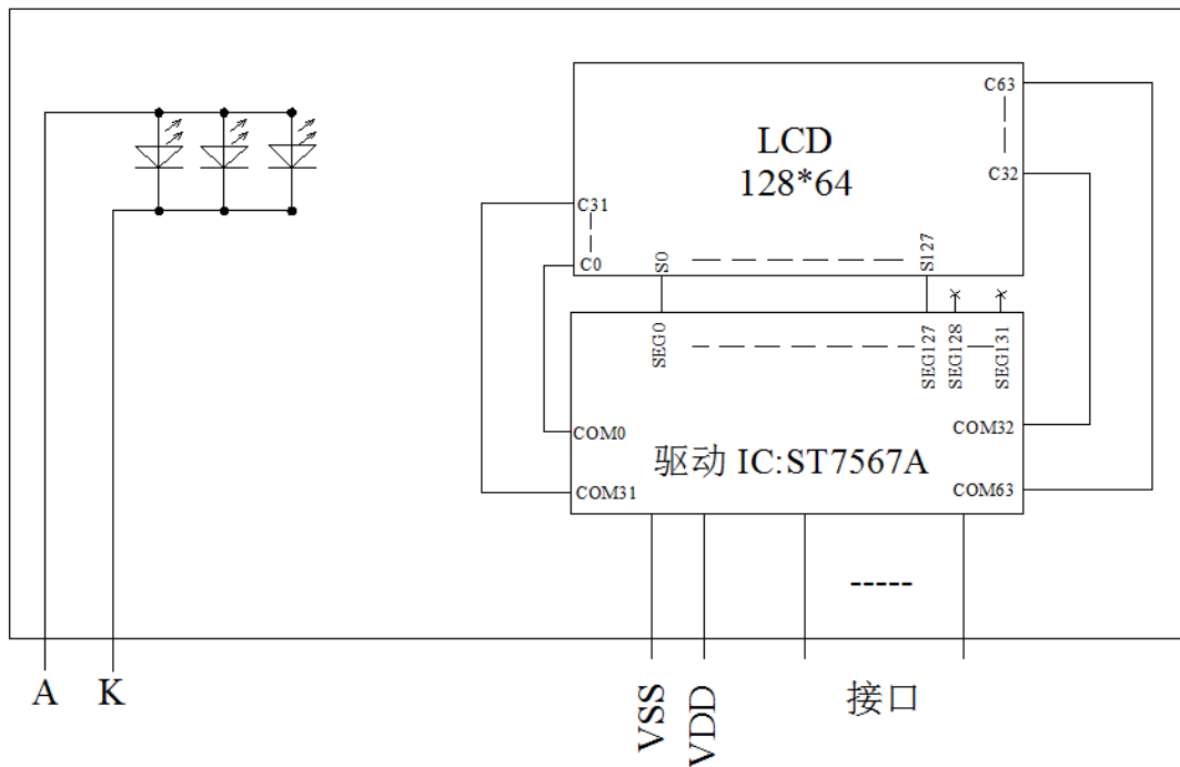
图 2: JLX12864G-21102 图像点阵型液晶模块的电路框图
