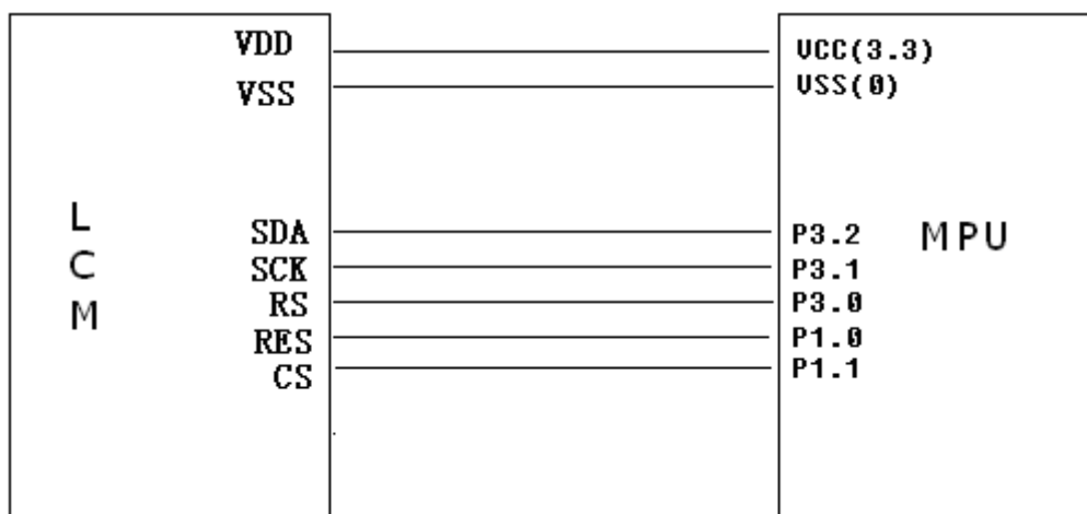
图 8. 串行接口
