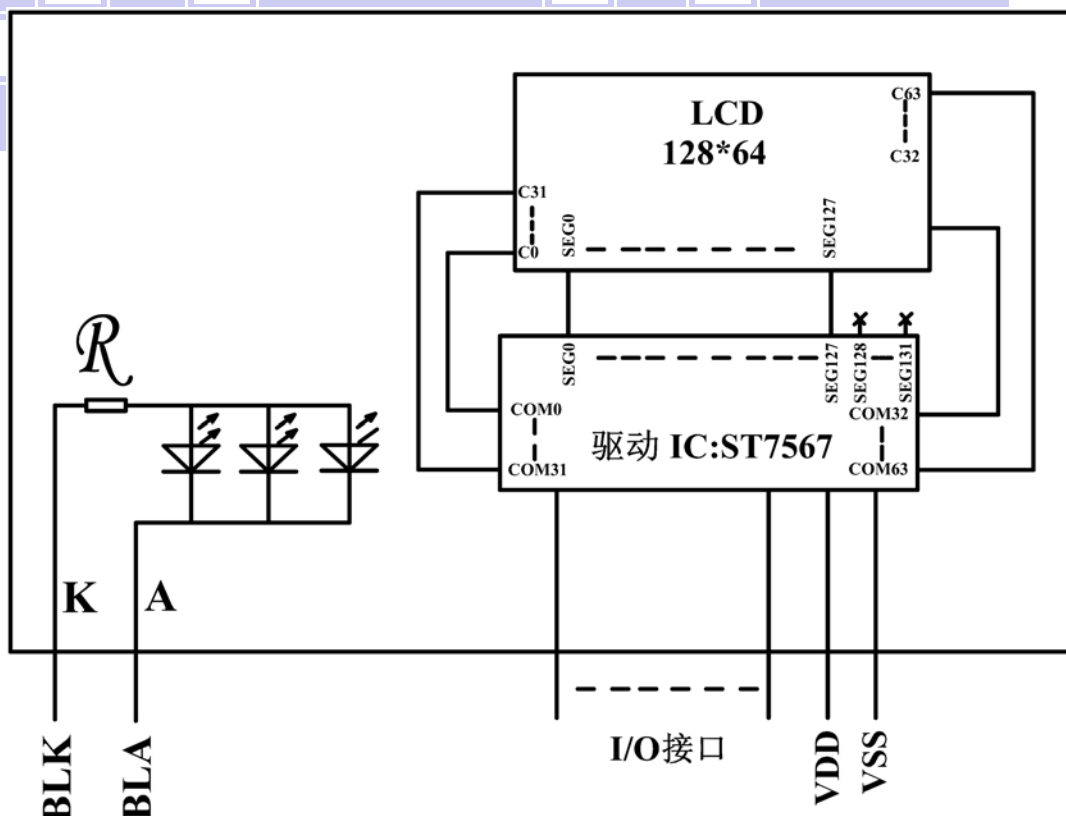
图 2: JLX12864G-33508-PN 图像点阵型液晶模块的电路框图
