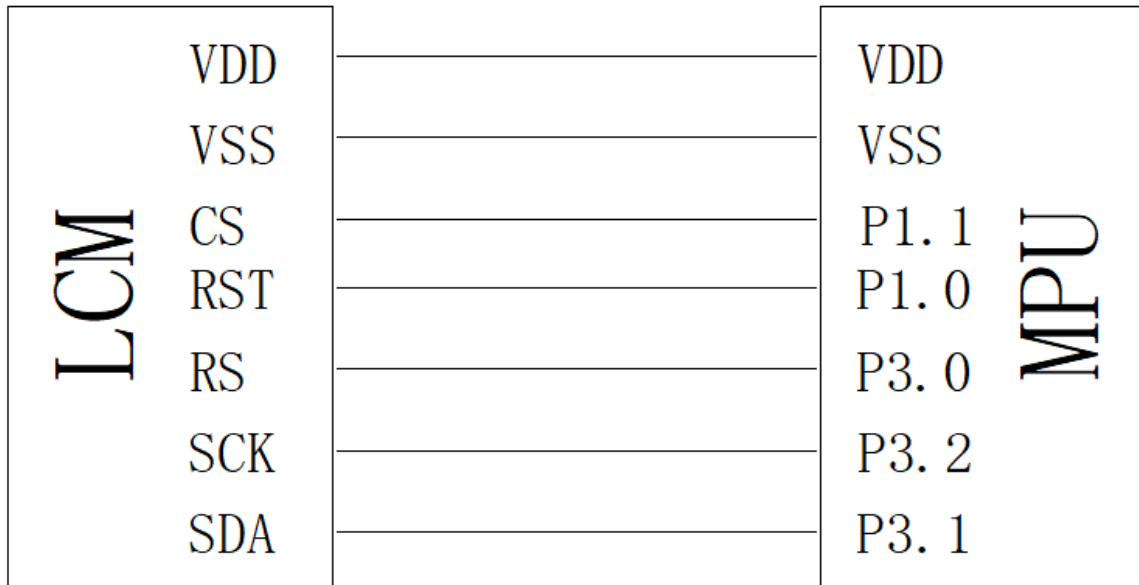
图 8. 串行接口
