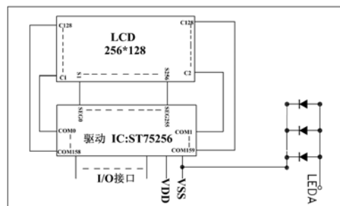
图 2: JLX256128G-978-PN 图像点阵型液晶模块的电路框图
