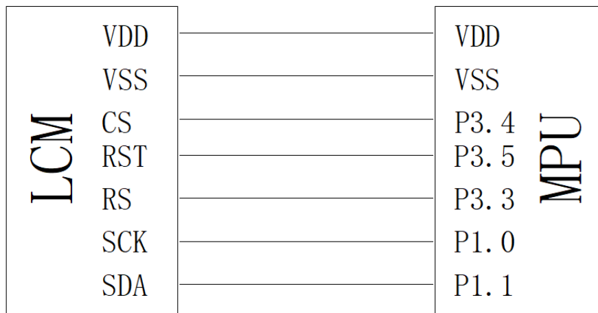
图 9. 串行接口
