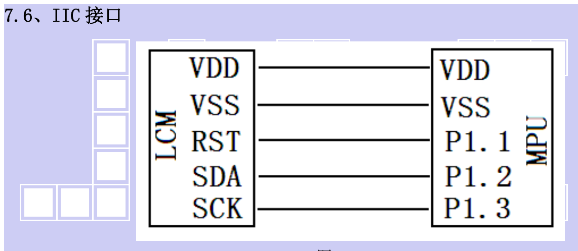
图 10. IIC
