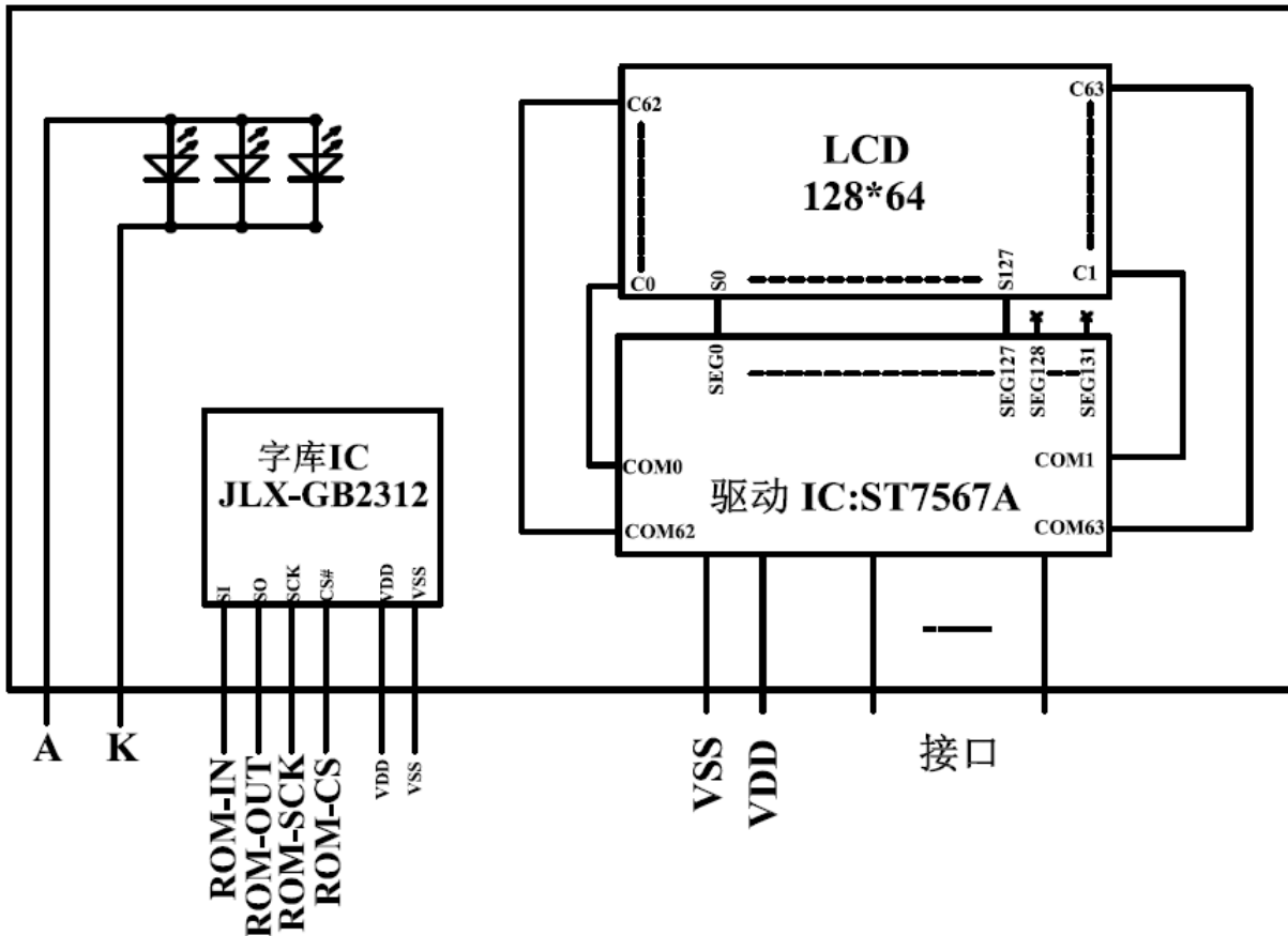
图 2: 电路框图
